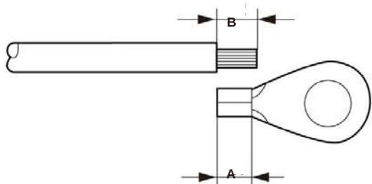
Figura 5.8 Lunghezza adatta
