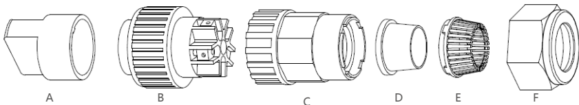
Figura 5.19 Connettore CA
