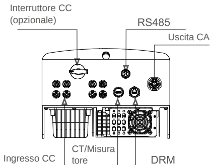
Figura 1.2 Vista dal basso
