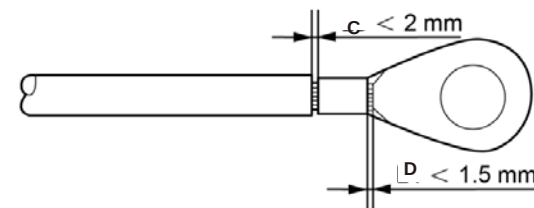
Figura 5.9 Cavo spellato
