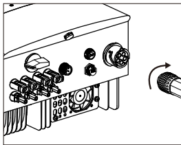
Figura 5.24: Collegamento all'inverter del connettore CA
