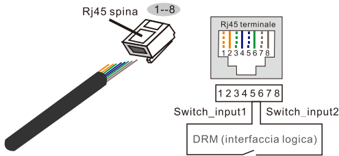
Figura 5.30 Spelare lo strato isolante e connettere alla spina RJ45
