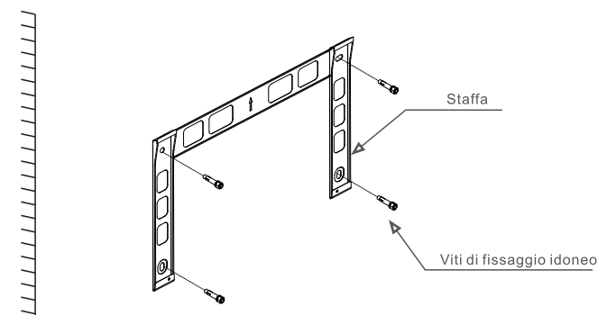
Figura 5.4 Montaggio a muro dell'Inverter
