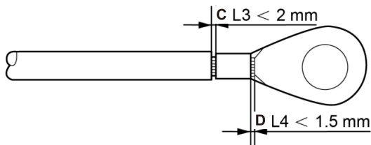
Figura.8 Spogliatura del cavo
