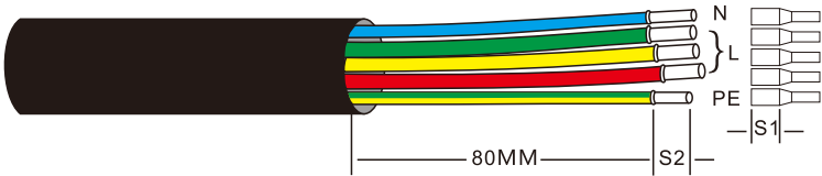
Figura 5.18 Cavo AC tolto
