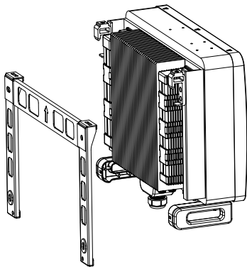
Figura 5.5 Installazione dell'inverter
