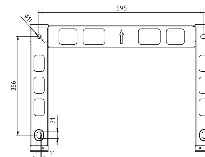
Figura 5.3 Montaggio a muro dell'Inverter
