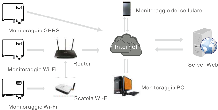
Figura 5.20 Funzione di comunicazione senza fili
