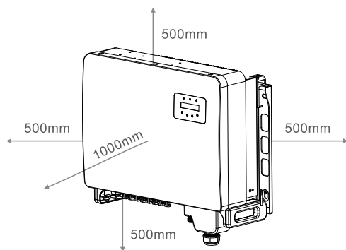
Figura 5.2 Spaziatura per Montaggio dell'Inverter
