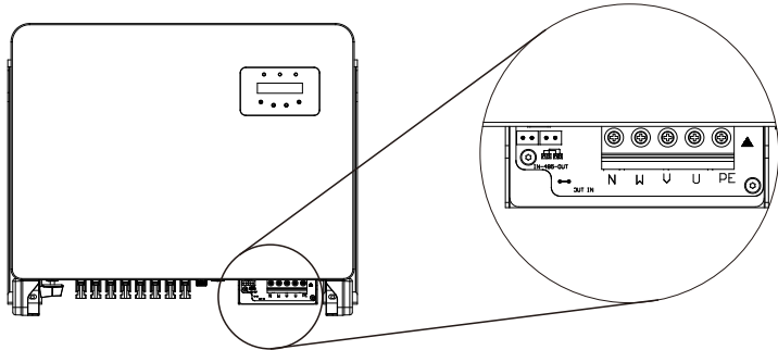
Figura 5.19 Cablaggio
